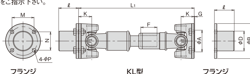
■KL型寸法表
